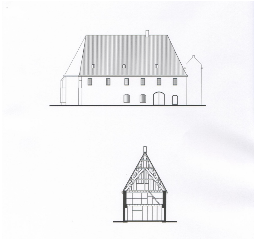
De situatie in 1857: Magazijn op den Uilenburg vooraanzicht en doorsnee (tekeningen Leo Sluijmer, arch. BNA)
