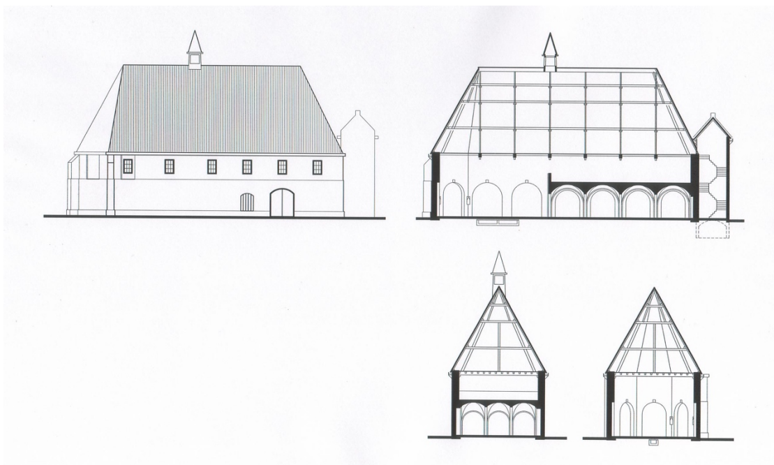
Reconstructie van de oorspronkelijke kloosterkapel. (Leo Sluijmer, architect BNA, 2005)
